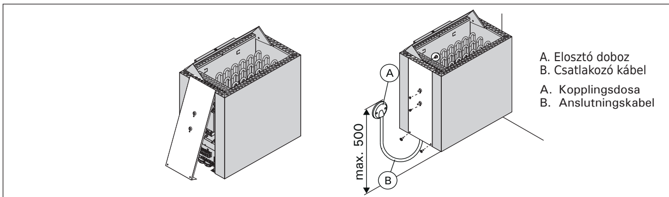
8. ábra. A csatlakozó doboz burkolatának lezárása (minden méret milliméterben értendő) Bild 8. Stänga anslutningshusets front (mått i millimeter)
