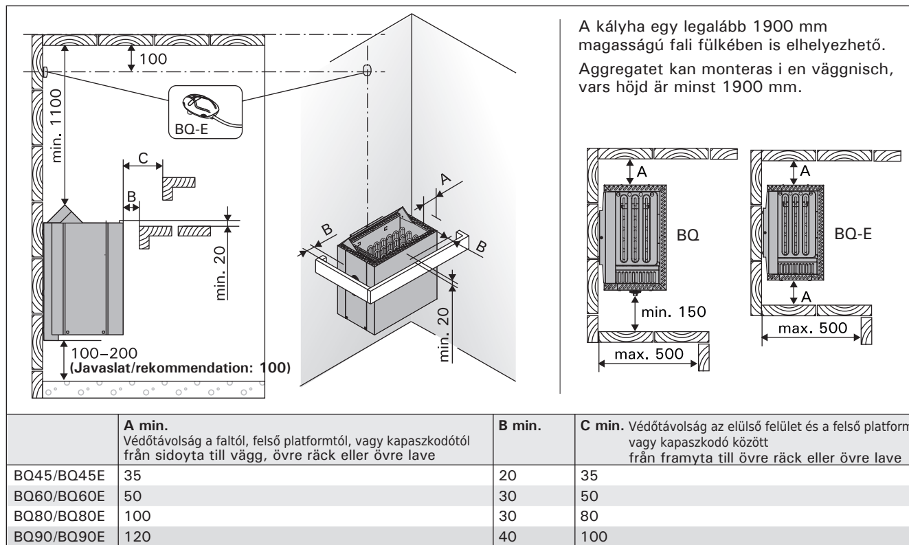
6. ábra Védőtávolságok (minden méret milliméterben értendő) Bild 6. Säkerhetsavstånd (mått i millimeter)
