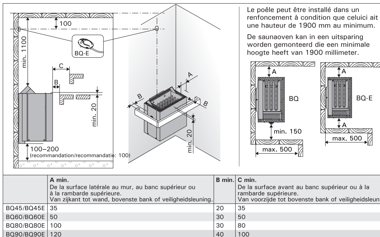
Figure 6. Distances de sécurité (toutes les dimensions sont fournies en millimètres)
