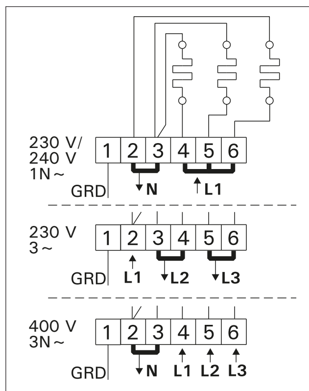
Figure 11. Raccordements électriques du poêle (BQ-E) Figuur 11. Elektrische aansluitingen (BQ-E)
