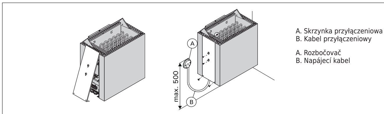
Rys. 8. Zamykanie pokrywy skrzynki przyłączeniowej (wymiały w milimetrach)
